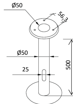
Art. 206ZZ Ancrage pour sol meuble Acier galvanisé
