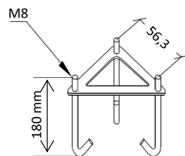
Art. 205ZZ Ancrage pour béton Acier galvanisé
