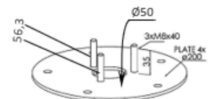
Art. 3080 Semelle de fixation pour sol dur Acier galvanisé 3080GA
