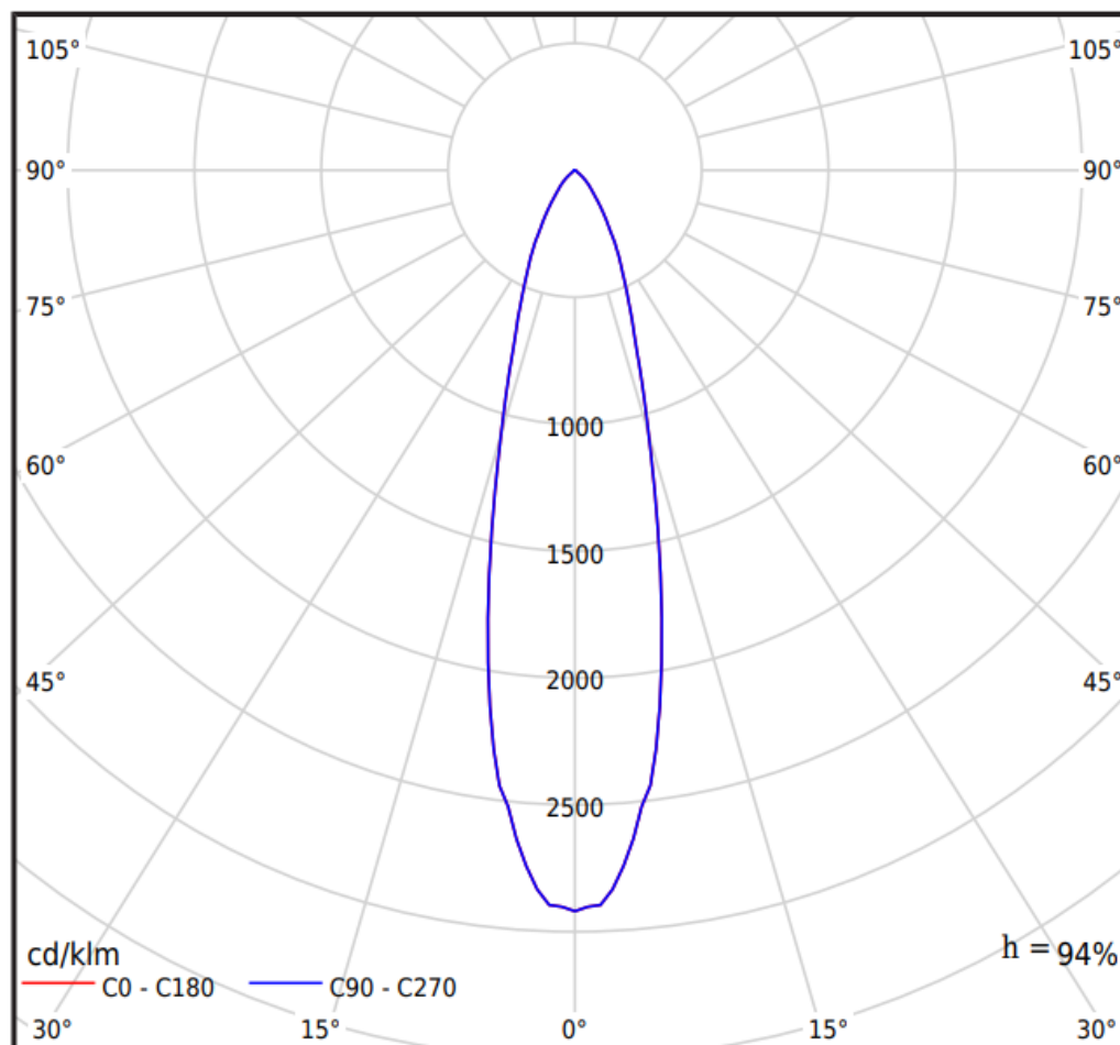
Schéma courbes photométriques pour art. 1373 :
