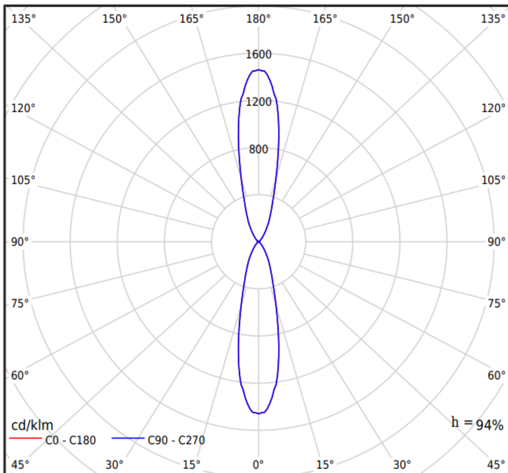
Schéma courbes photométriques pour art. 1370 :
