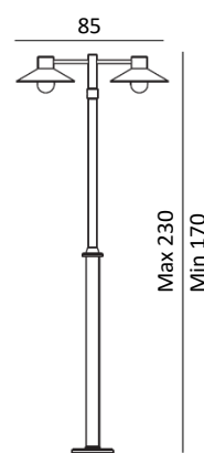
Art. 275 E27, 2x57W Halo. max. Energieklasse: A bis G Verzinkt 275GA Schwarz 275SV
