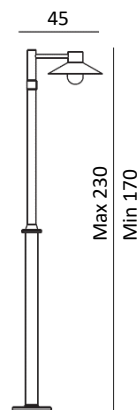
Art. 274 E27, 57W Halo. max. Energieklasse: A bis G Verzinkt 274GA Schwarz 274SV
