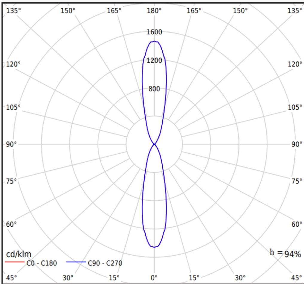
Diagramm der photometrischen Kurven für Art. 1370:
