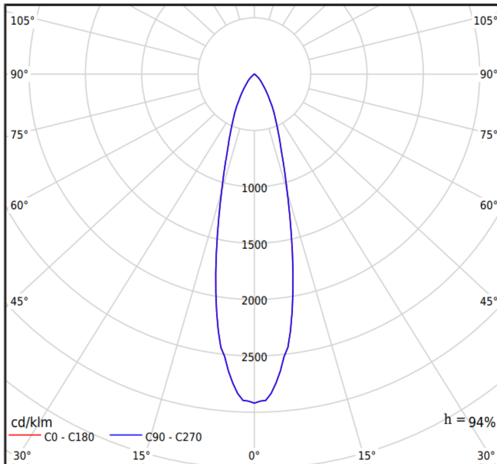
Diagramm der photometrischen Kurven für Art. 1373:
